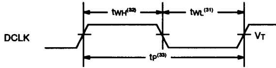
DCLK Width/Period
